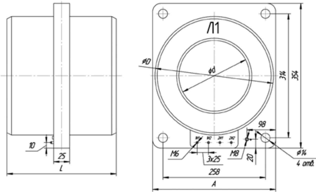
ГАБАРИТНЫЕ, ПРИСОЕДИНИТЕЛЬНЫЕ, УСТАНОВОЧНЫЕ РАЗМЕРЫ И МАССА ТРАНСФОРМАТОРОВ ТОКА
