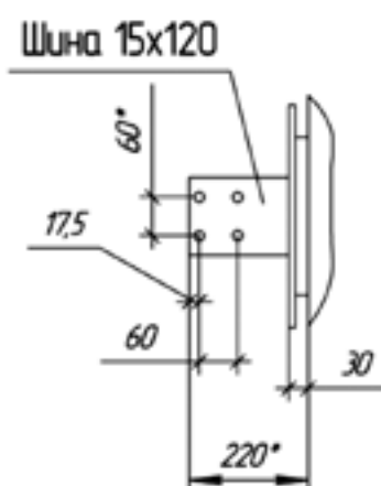
Страна НН ТМЗ-2500
