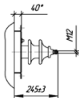
Б Страна ВН ТМЗ-250-2500
